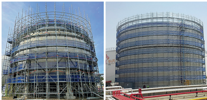
(주)디아엔지니어링의 원형 시스템 비계. 세계 최초로 개발돼 현장에 적용된 볼 탱크(Ball Tank) 전용 시스템 비계이다.
